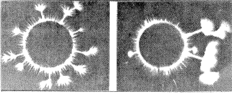
شكل ( ١٠ أ ) يوضح كيف يتأثر التصوير الكيرلياني بالفازات المختلفة ، فيعطي أشكالاً متباينة لقرص معدني السلي المهيمن عليه خليط من غازي النيتروجين ورابع كلوريد الكربون ونفس القرص المي إلى اليسار وعليه غاز الفريون . . لاحظ كيف تختلف الهالة بين هذا وذاك .
